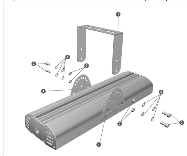
Рисунок 3. Схема монтажа светильника GSFNO на поворотное крепление.
