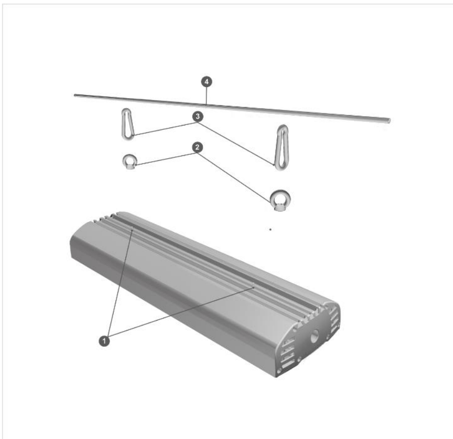
Рисунок 1. Схема монтажа светильника GSFNO на подвесное крепление.
